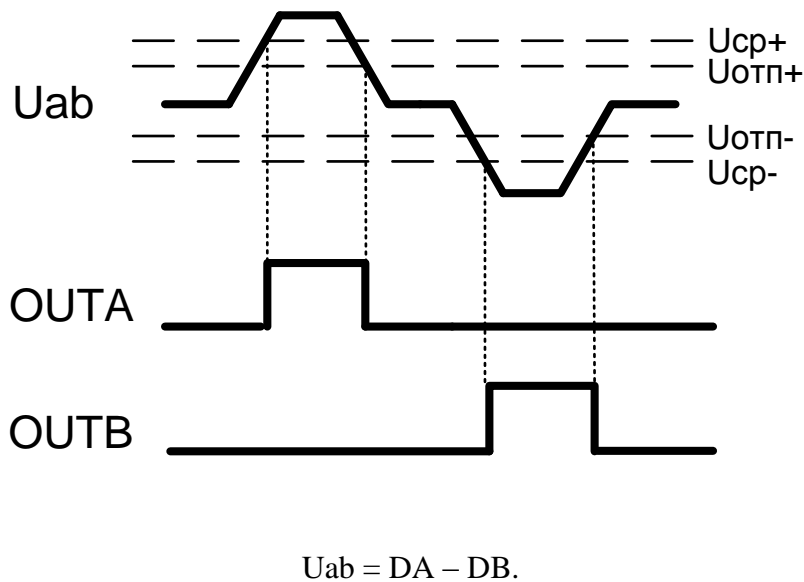
Р и с у н о к 2.1 – Диаграмма срабатывания выходных сигналов микросхем относительно разницы сигналов между входами DA и DB
